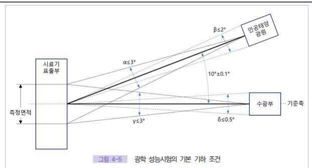
그림 4-5 광학 성능시험의 기하 조건
