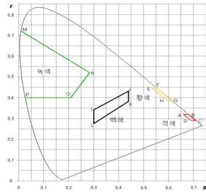
그림 4-3 색도도
