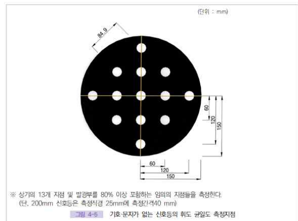
그림 4-5 기호·문자가 없는 신호등의 휘도 균일도 측정지점
