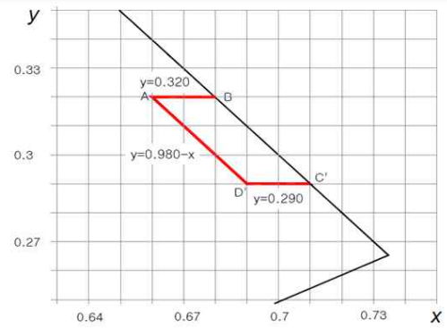
그림 4-4 적색 범위도
