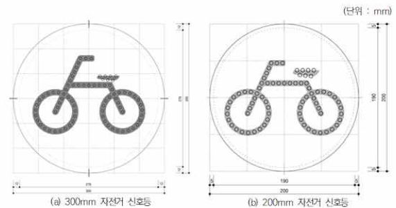
그림 4-5 자전거 신호등 형상
