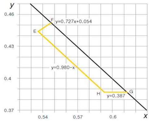
그림 4-5 황색 범위도
