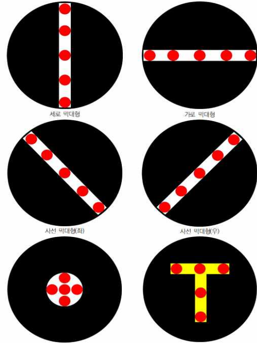
그림 4-5 노면전자 신호등의 휘도 균일도 측정지점
