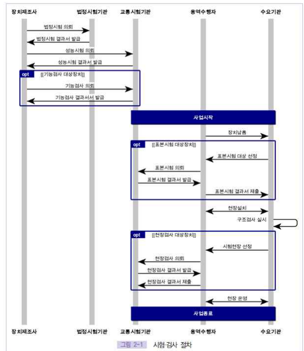
그림 2-1 시험·검사 절차
