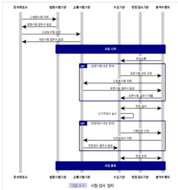
그림 2-1 시험·검사 절차
