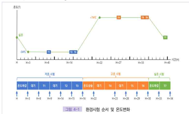
그림 4-1 환경시험 순서 및 온도변화
